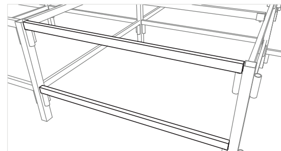
ELEMENTO LONGITUDINAL
